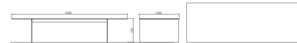
Size : W3500×D1200×H720mm
