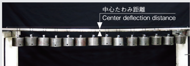
25φ Mフリーパイプ 25φ M Free Pipe L: 1500mm(4.92')
