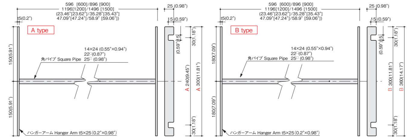
ハンガーアーム t5 × 25 Hanger Arm 15×25(0.2"×0.98") A P240×D300(9.45"×11.81") B P300×D360(11.81"×14.17")
